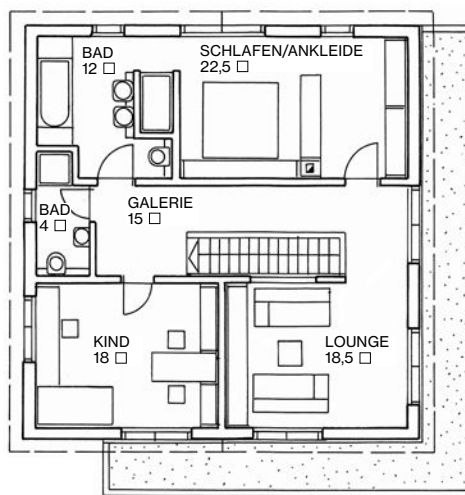
OBERGESCHOSS
